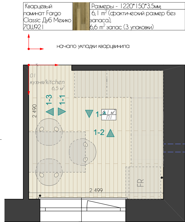
план полов М 1:35
