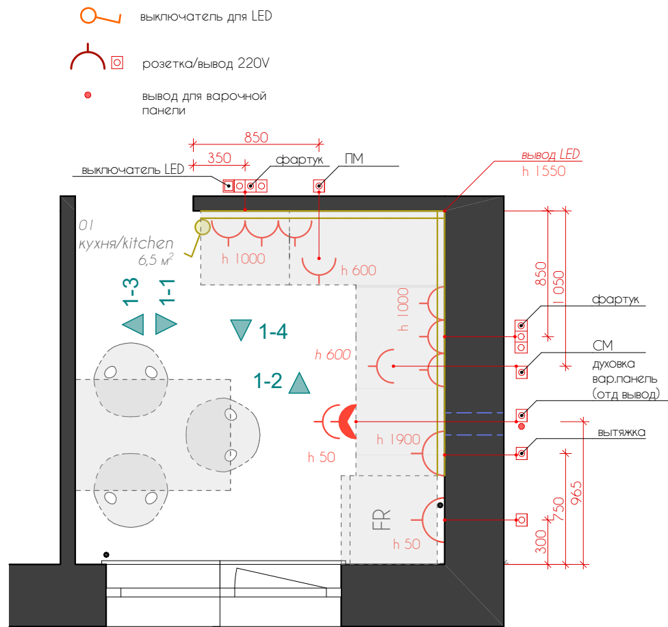
план электрооборудования М 1:35
